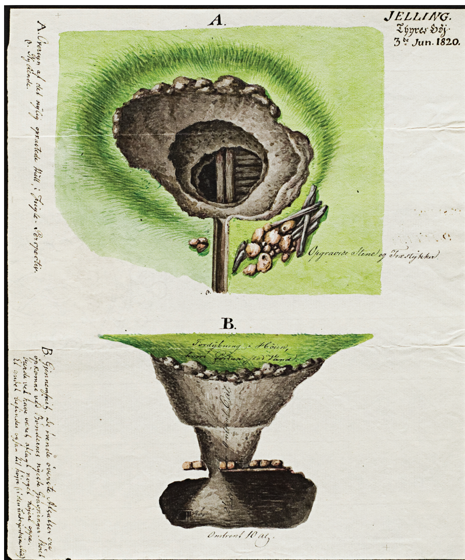
Fig. 2. Plan og snit (set mod syd) af gravningen i Nordhøjen, udført af bønderne i Jelling i 1820. Akvarel: J.H.T. Hanck, Nationalmuseet.
